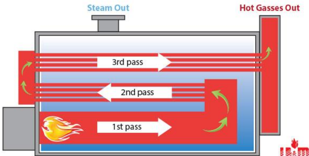
دیگ بخار سه پاس
